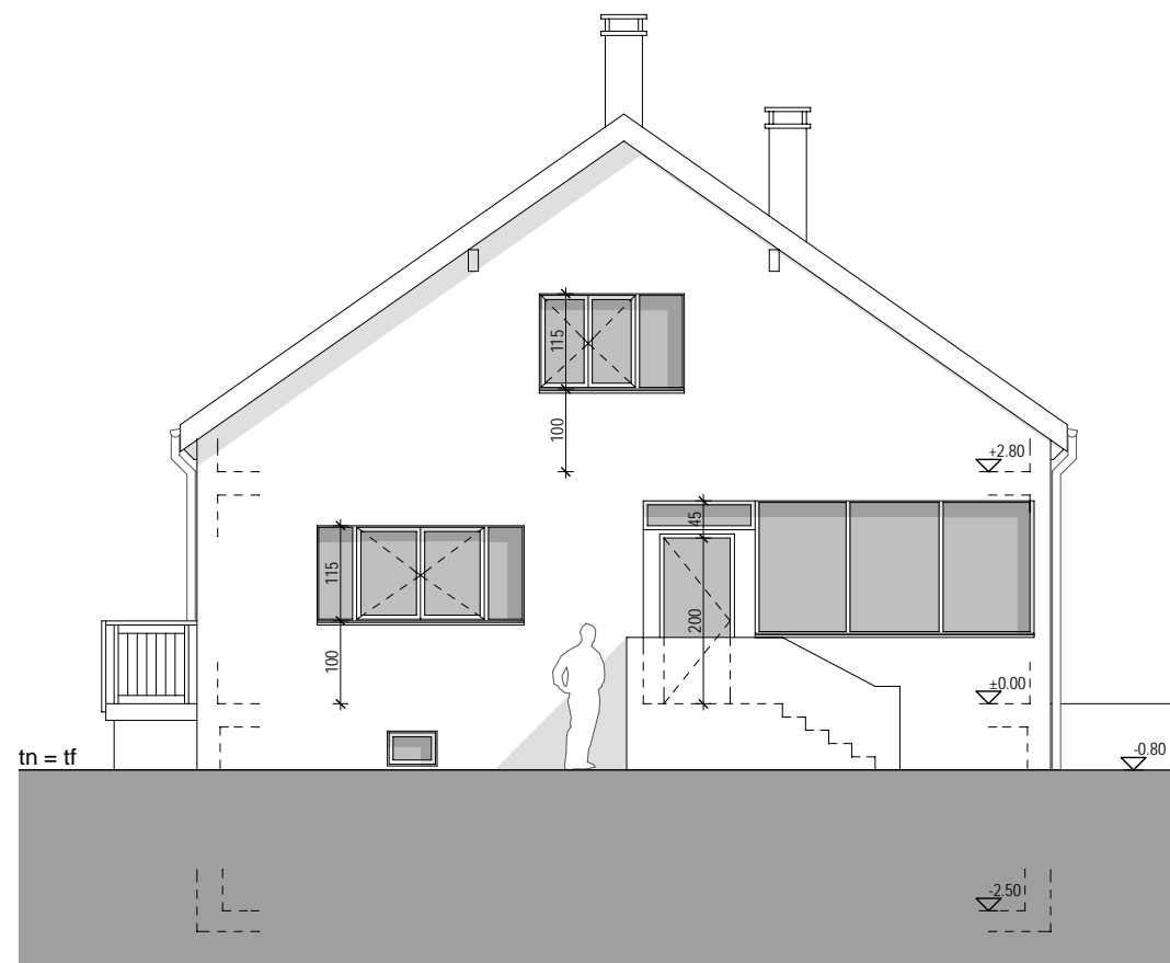
Façade Sud
